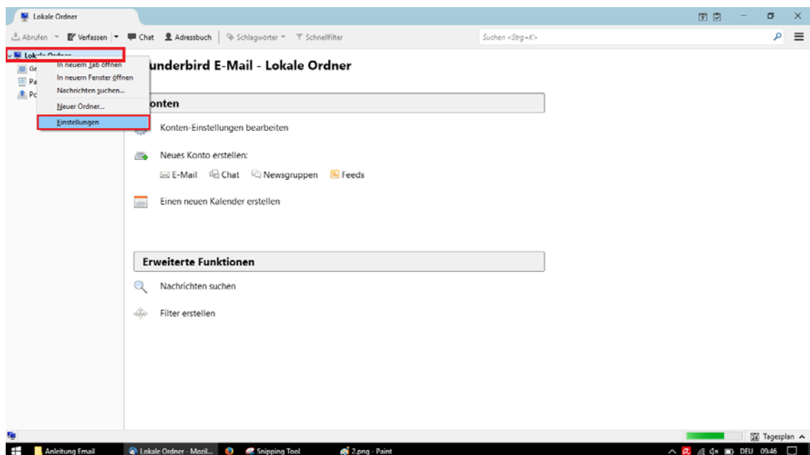
Abbildung 1: E-Mail-Programm
