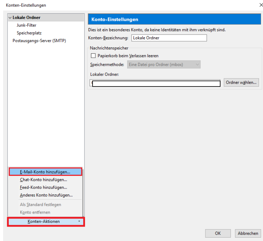
Abbildung 2: Konto-Einstellungen
