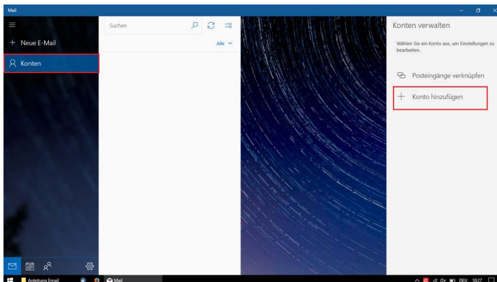
Abbildung 1: E-Mail-Programm
