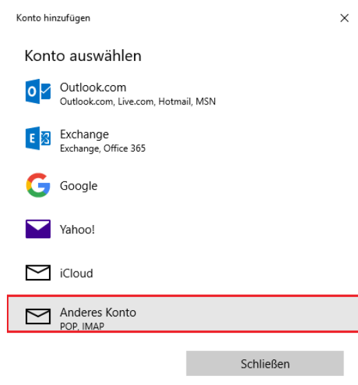
Abbildung 2: Konto hinzufügen
