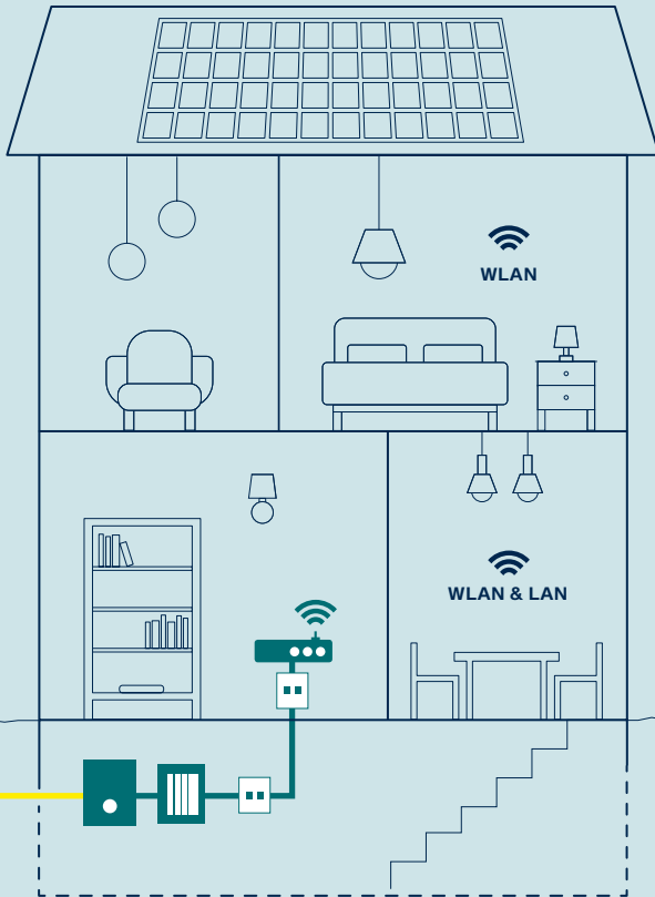
Beispiel für eine Netzwerkverkabelung
